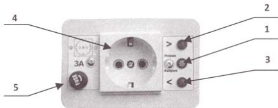
Рис.2 Стабилизатор (вид на лицевую панель)
