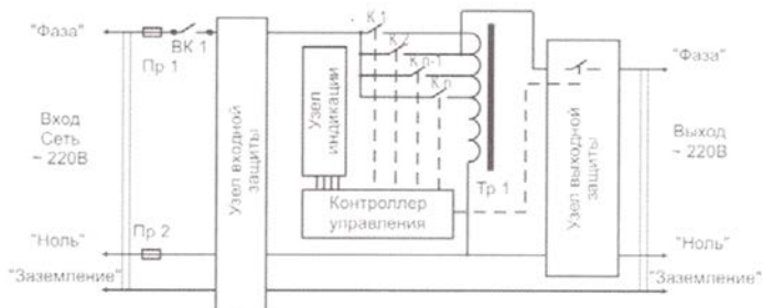
Рис.1 Функциональная схема
